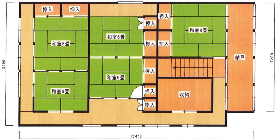
2階平面図
